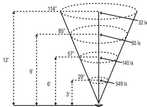
LPAR36-LED-8W-WF
