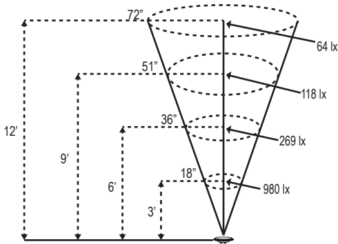
LPAR36-LED-4W-F
