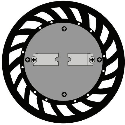
LPAR36-LED-4W-F
