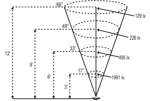
LPAR36-LED-10W-F
